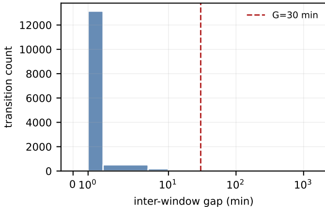
GeoLife
