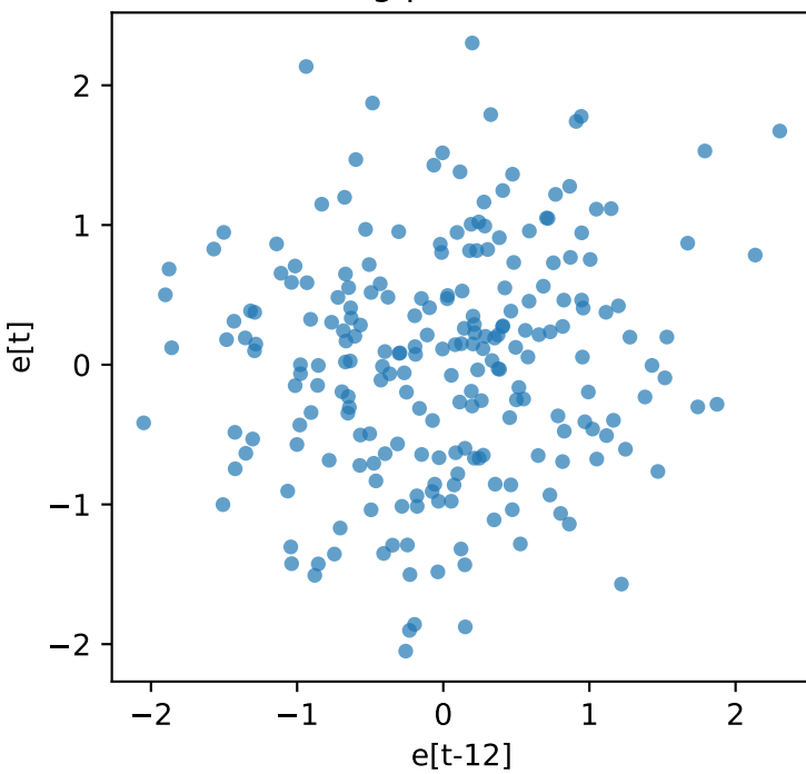
Lag plot, h=12
