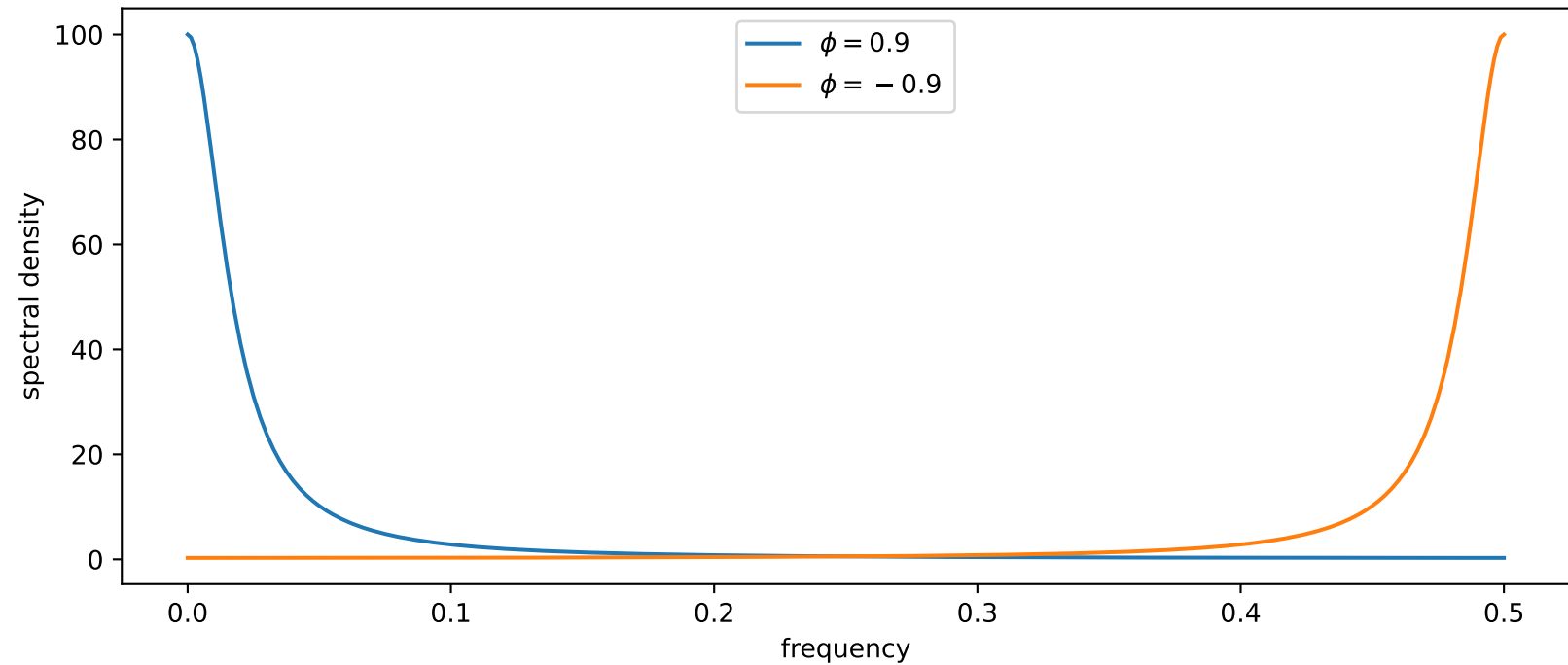
AR(1) spectra
