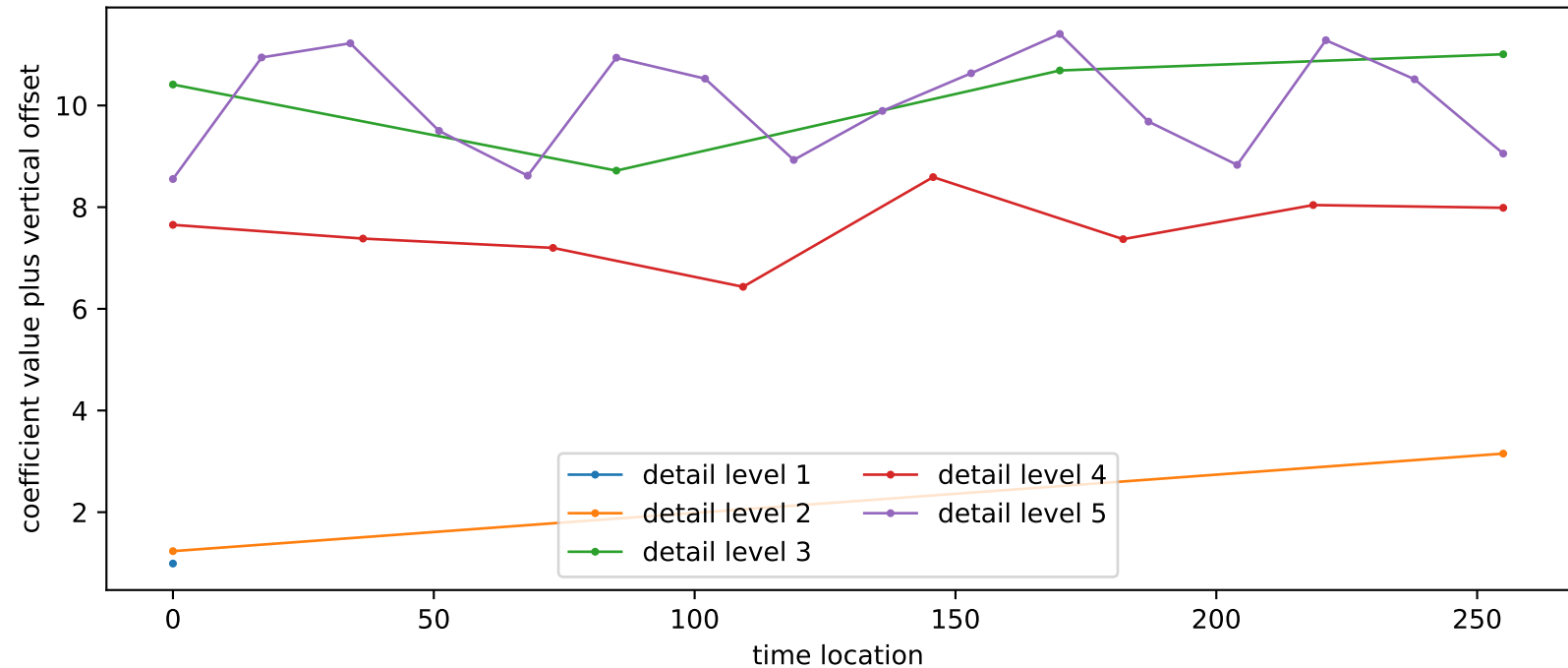
Multiscale Haar detail coefficients
