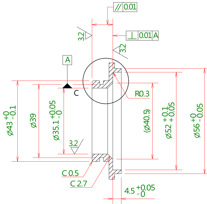
B-B(1:1)
