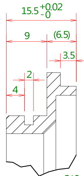
C(2:1)
