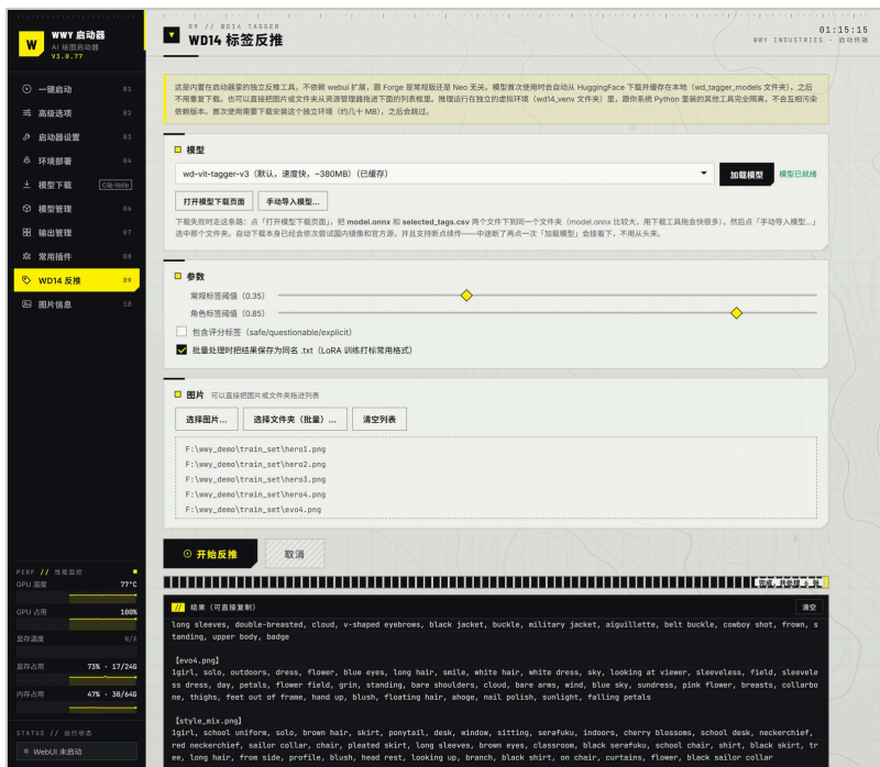
图 WD14 反推实际运行结果：6 张图批量打标，每张图旁边生成了同名 .txt。
