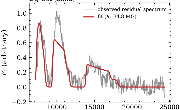
EQ Cet (blind)
