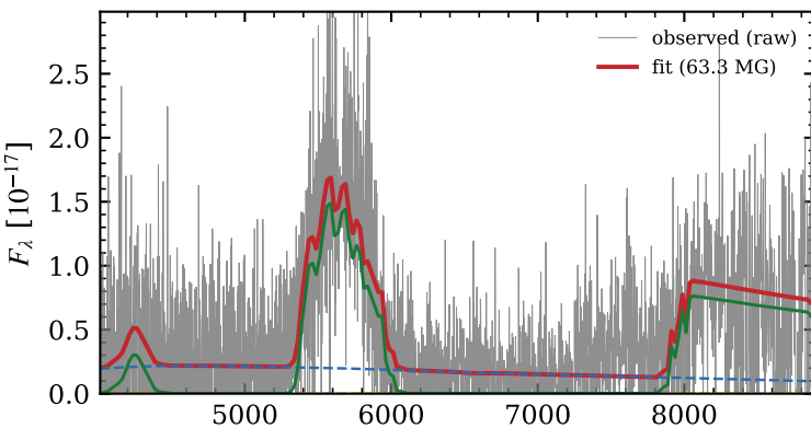
PZ Vir
