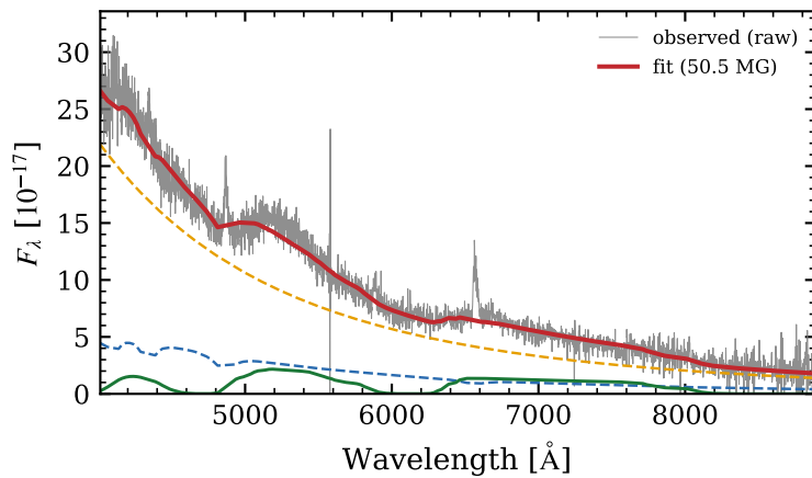
SDSS J1344+2044
