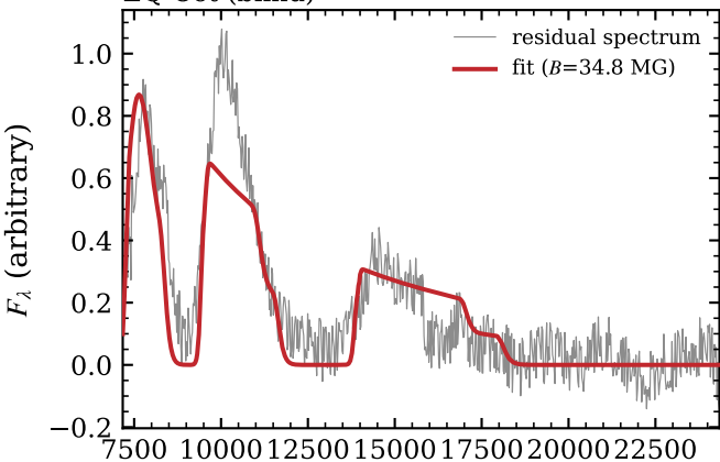
EQ Cet (blind)
