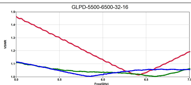
VSWR
