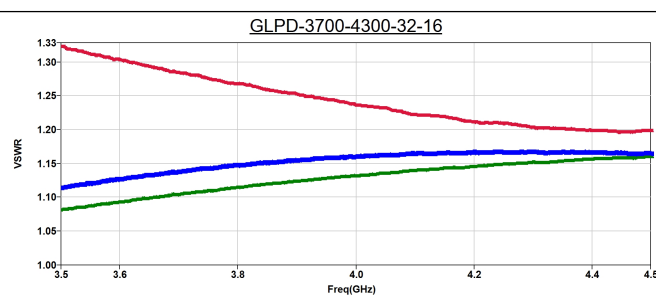
VSWR
