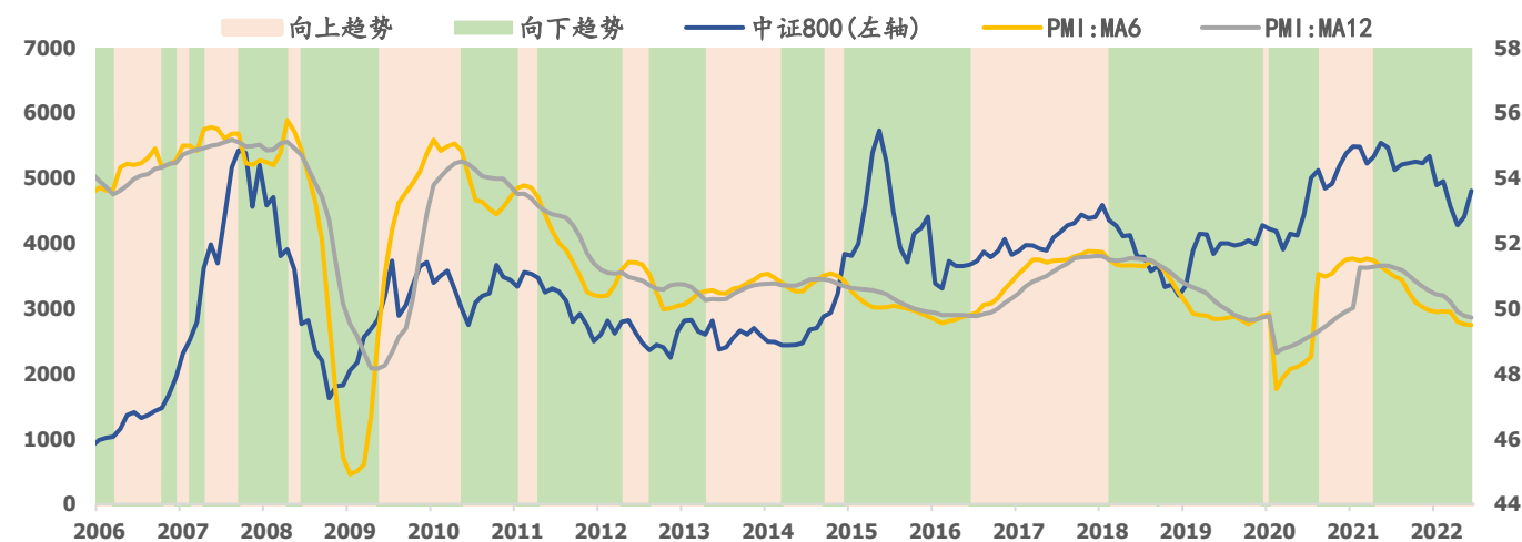
图表 8: PMI
