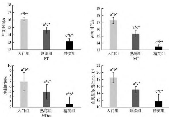
图3 三组受试者羽毛球专项RSA测试对比
