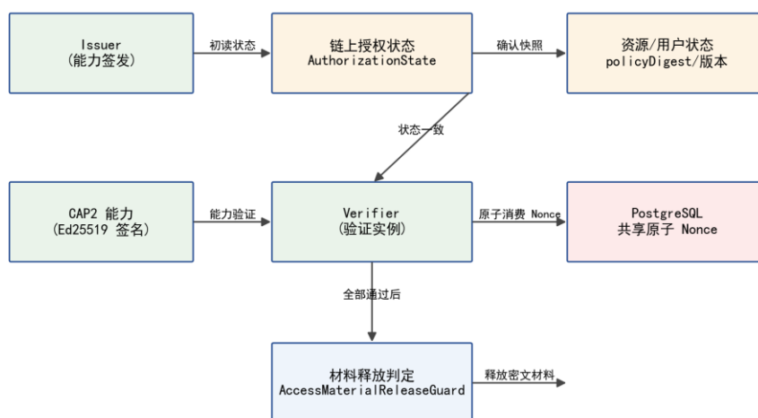
图 CAP2 能力签发与验证流程（依据冻结协议绘制）
