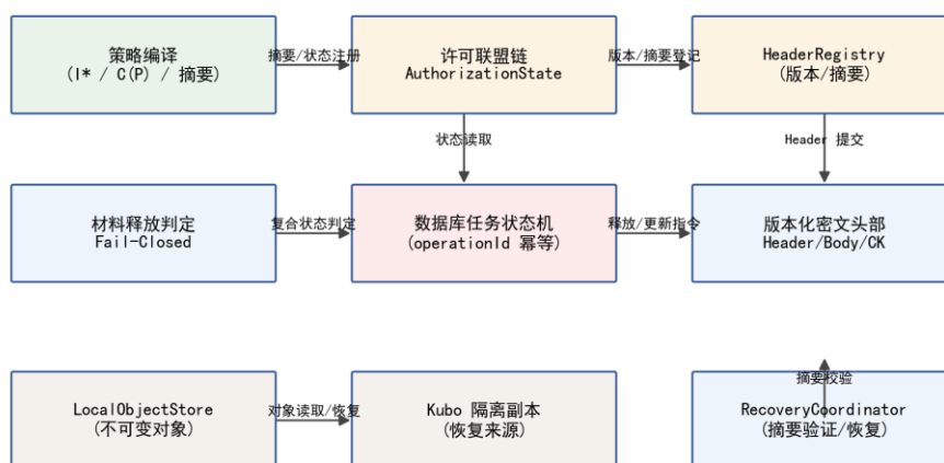
图 链上授权状态、任务状态与链下对象闭环架构（依据冻结方案绘制）
