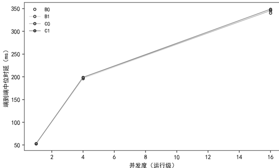
图 9 并发度对端到端时延的影响 (RC2)
