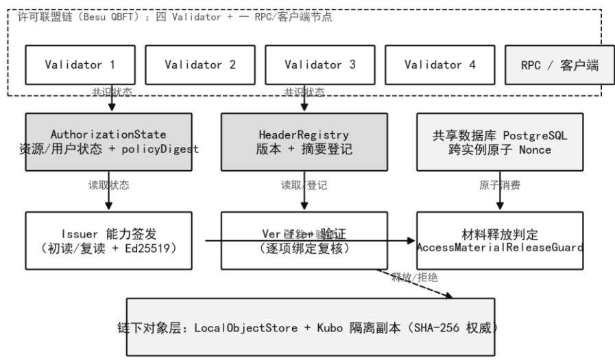
图 7 许可联盟链可信授权系统总体架构
