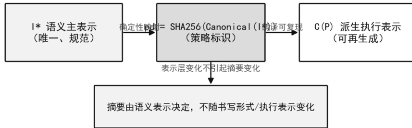
图 3 语义主表示—摘要—派生执行 IR 关系
