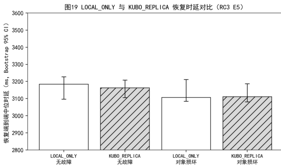
图 19 LOCAL_ONLY 与 KUBO_REPLICA 恢复时延对比 (RC3 E5)
