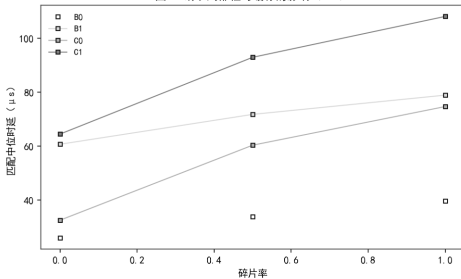
图 14 碎片率对匹配时延的影响 (RC2)
