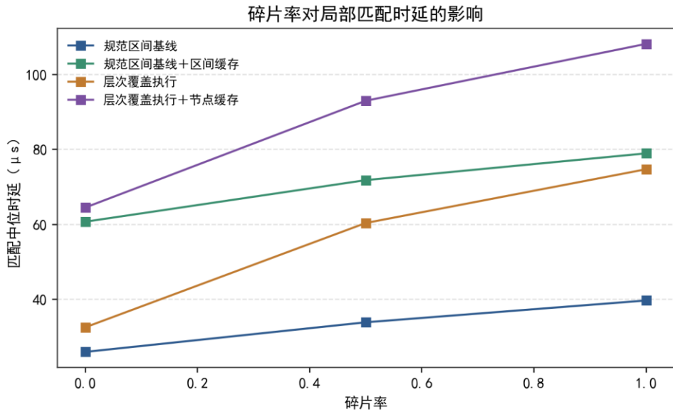
图 14 碎片率对匹配时延的影响（许可链可信授权实验）
