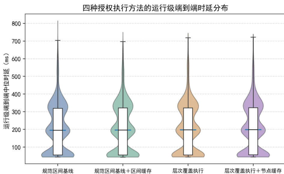
图 10 四种授权执行方法的运行级端到端时延分布（许可链可信授权实验）
