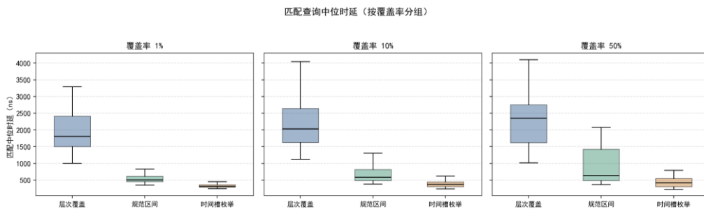
图 4 匹配查询中位时延（表示规模与查询开销实验）
