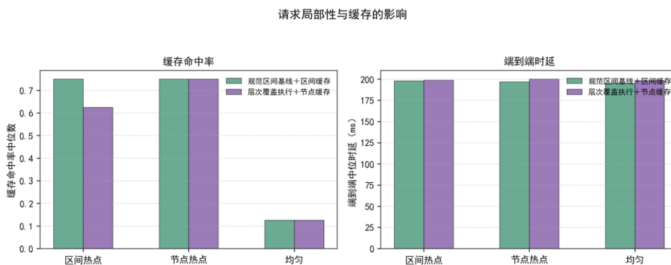
图 11 请求局部性与缓存的影响（许可链可信授权实验）
