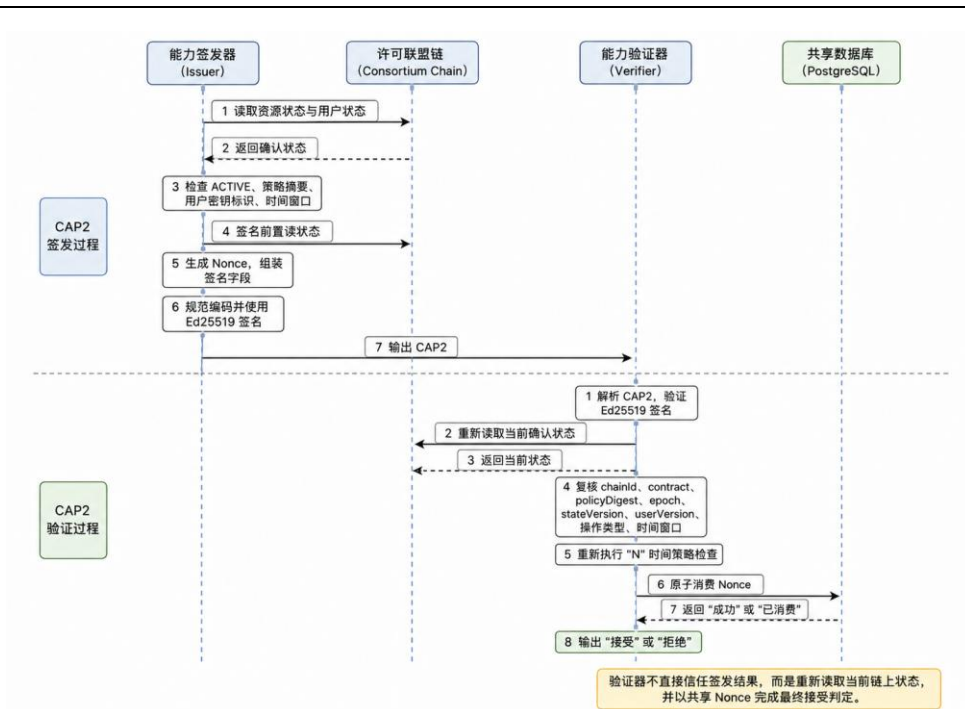
图 8 上下文完整绑定能力凭证签发与验证流程
