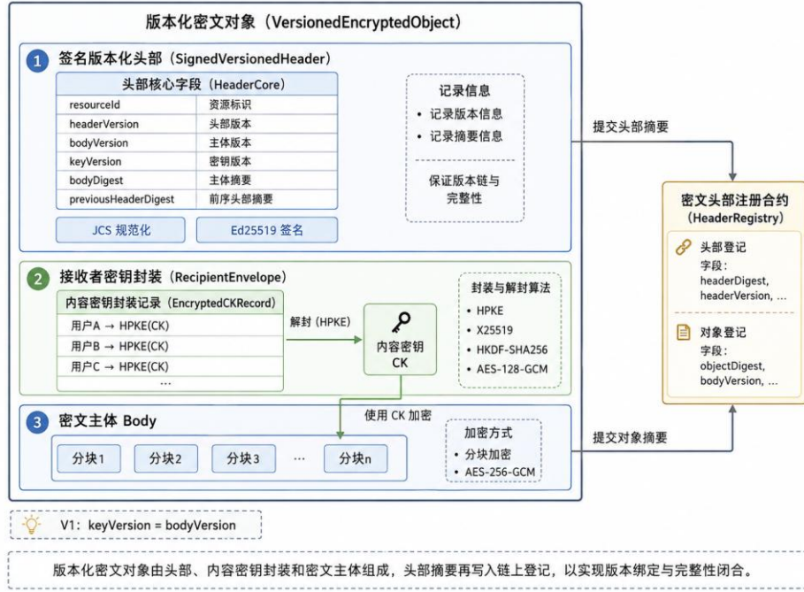
图 15 版本化密文对象结构（密文头部/密文主体/内容密钥）
