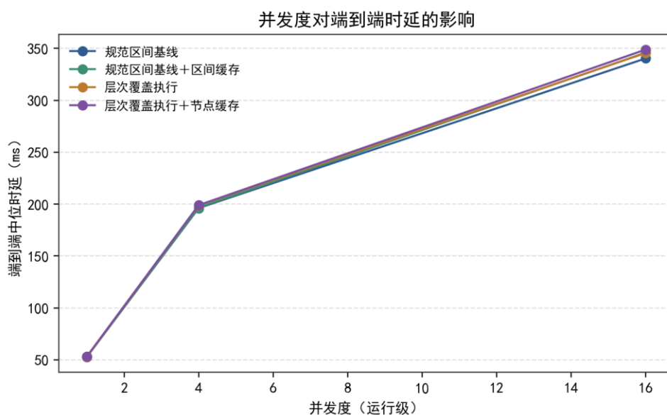
图 9 并发度对端到端时延的影响（许可链可信授权实验）
