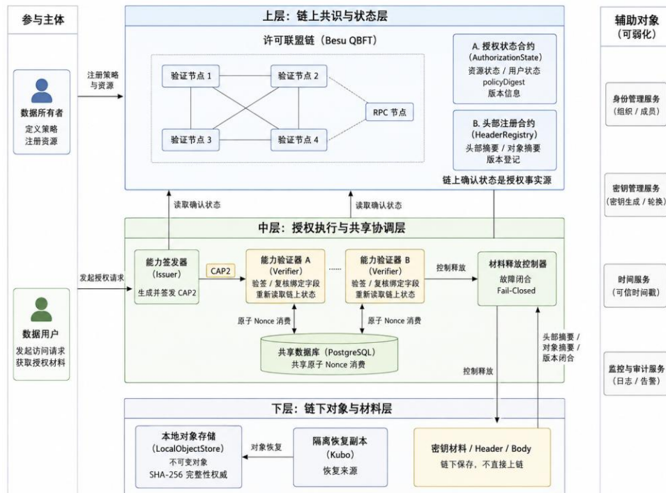
图 7 许可联盟链可信授权系统总体架构
