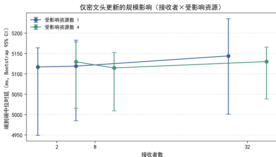
图 18 仅密文头更新的规模影响（接收者×受影响资源，版本化密文生命周期实验）
