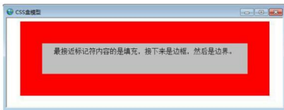
图 7.3 CSS 盒模型
