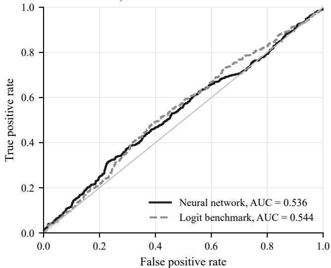
A. ROC curve, 2022-2023 holdout
