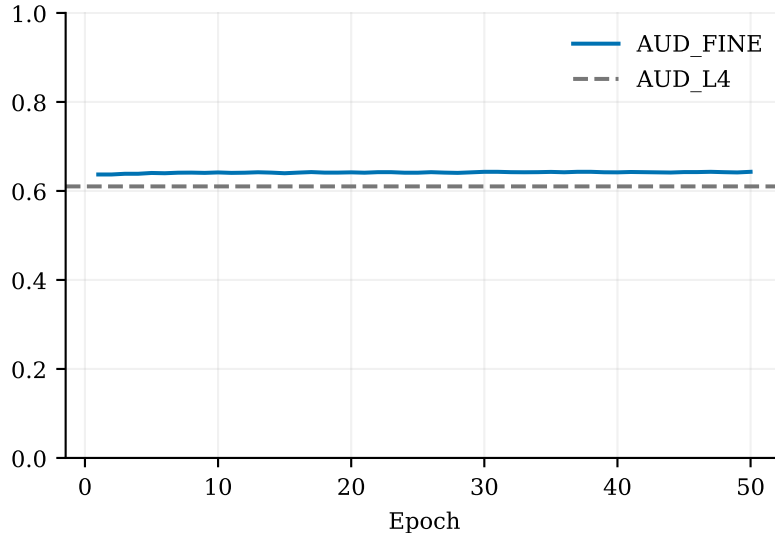
AUC
