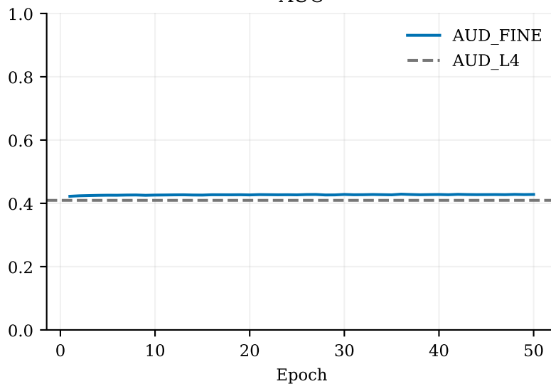
AUC
