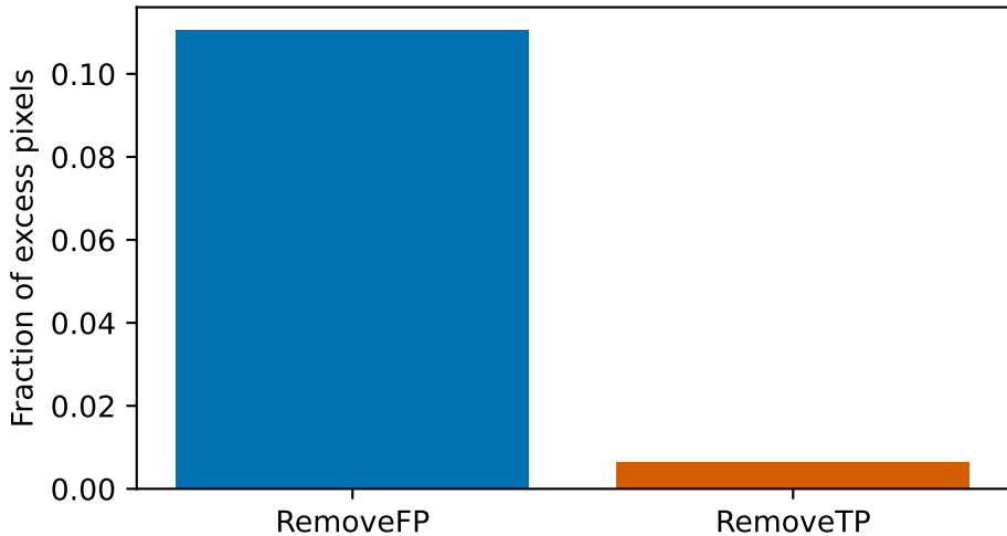
VGG Group-A
