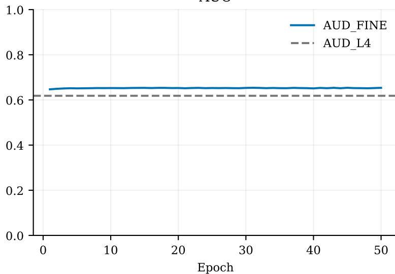
AUC
