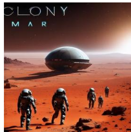
SD-3.5-M
