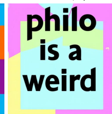
GRPO-Mix
