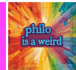
Ours
