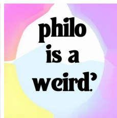
GRPO-OCR
