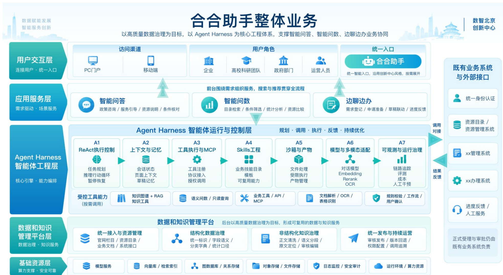
图 1 合合助手整体架构
