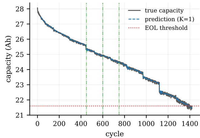
GOTION LFP · 27 Ah
