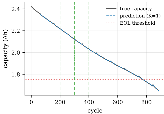
TJU (CY25-1) NCM+NCA · 2.5 Ah
