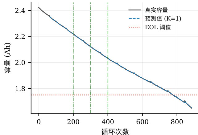
TJU (CY25-1) 三元 (NCM)+镍钴铝 (NCA) · 2.5 Ah
