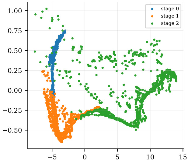
PCA projection
