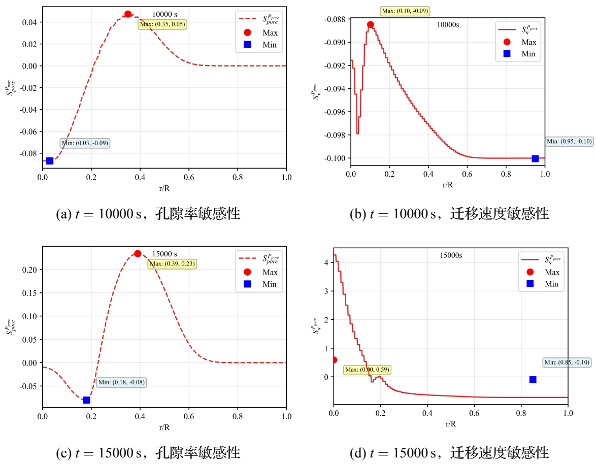
图 3-13 不同时间下气孔压力对孔隙率和气孔迁移速度的敏感性指标沿燃料半径方向的分布
