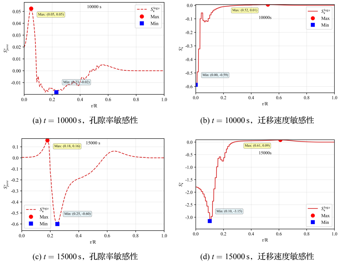
图 3-14 不同时间下人工扩散系数对孔隙率和气孔迁移速度的敏感性指标沿燃料半径方向的分布
