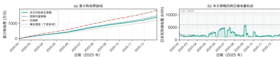
(b) 各策略累计费用与跨日储电量
