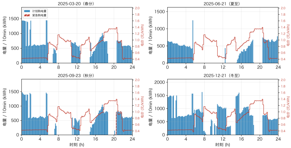
图 6 指定日期的计划购电量、紧急购电量与电价
