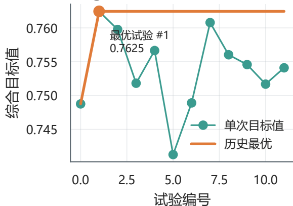
LightGBM 贝叶斯调参轨迹
