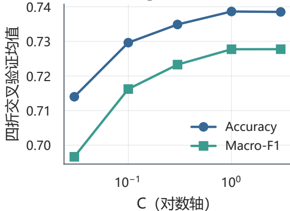
Ordinal Logistic 正则强度搜索
