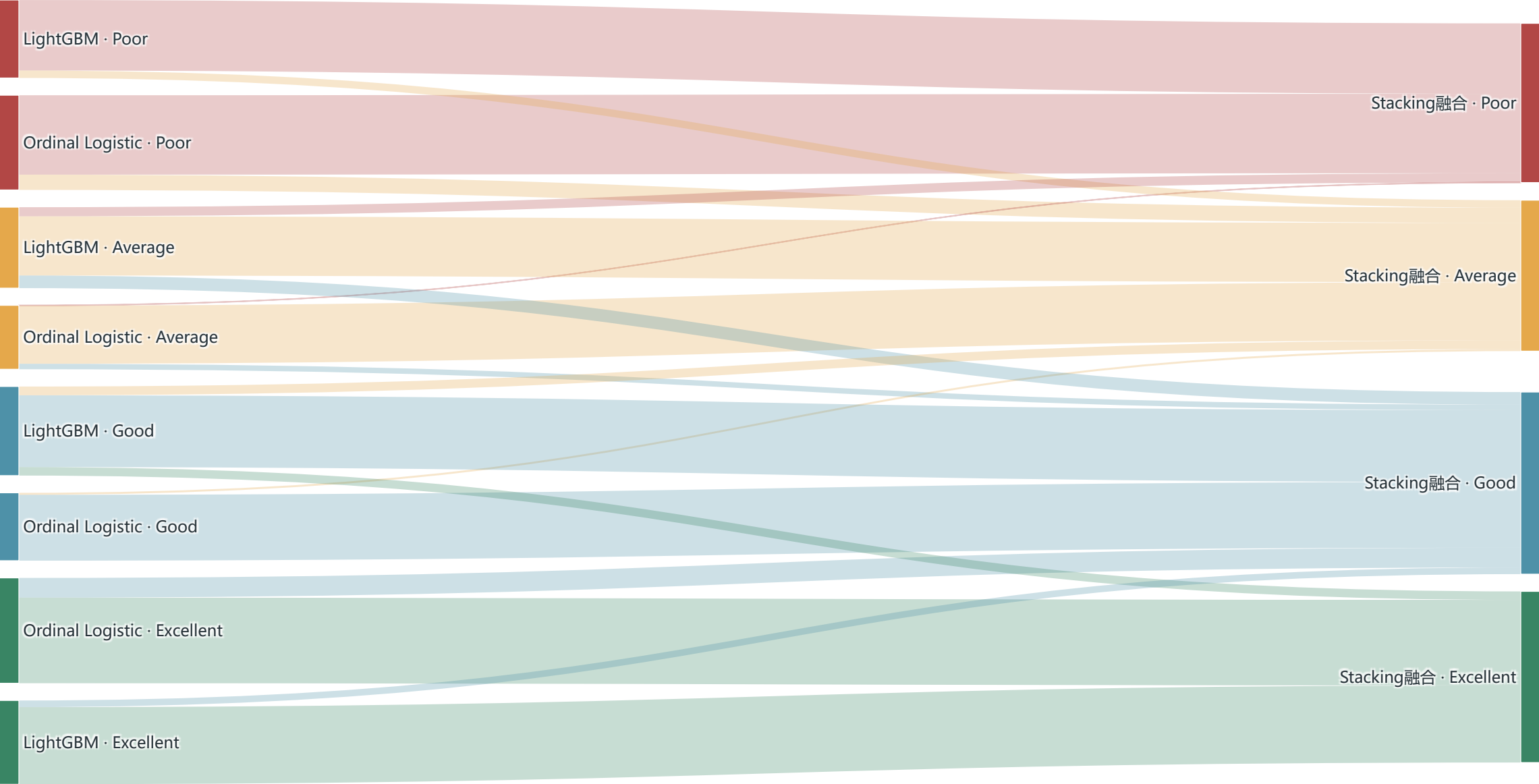
任务二一级模型预测等级到Stacking最终判断的流向
