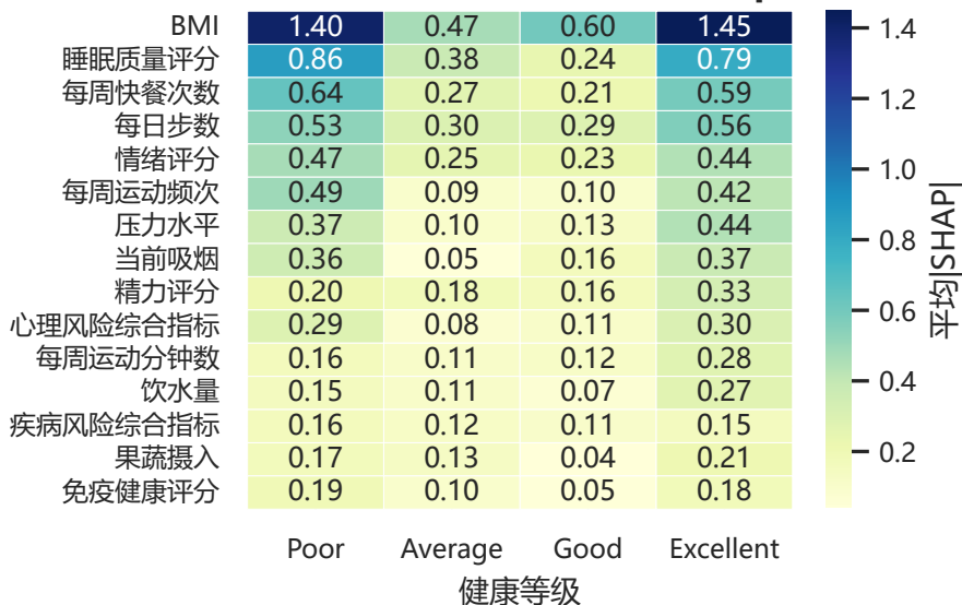
各等级全局SHAP重要性热力图 (Top 15)
