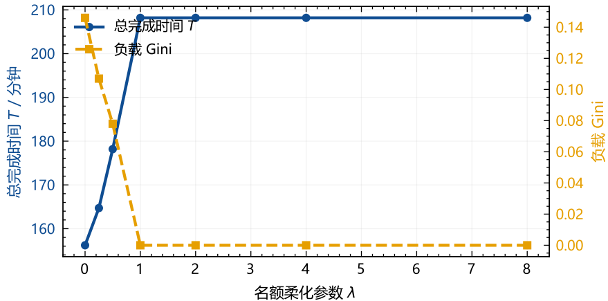
T 上升而 Gini 下降：两个目标不一致
