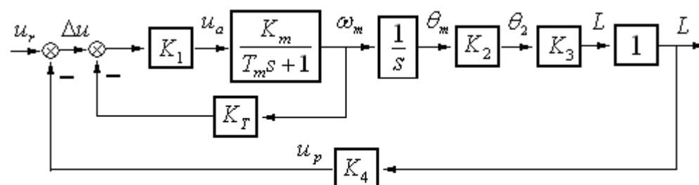
函数记录仪方框图
