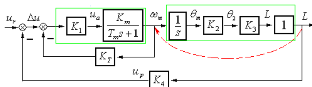
函数记录仪方框图
