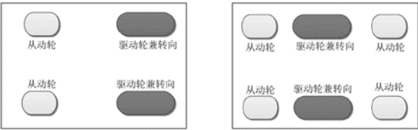
图 2-2 差速驱动示意图
