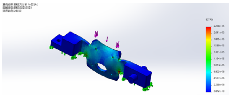
图 3-6 支撑梁应变最大分布示意图
