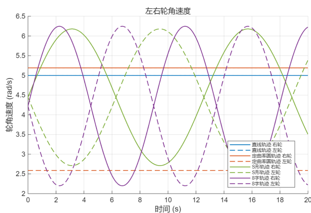
图 5-8 四类轨迹左右轮角速度
