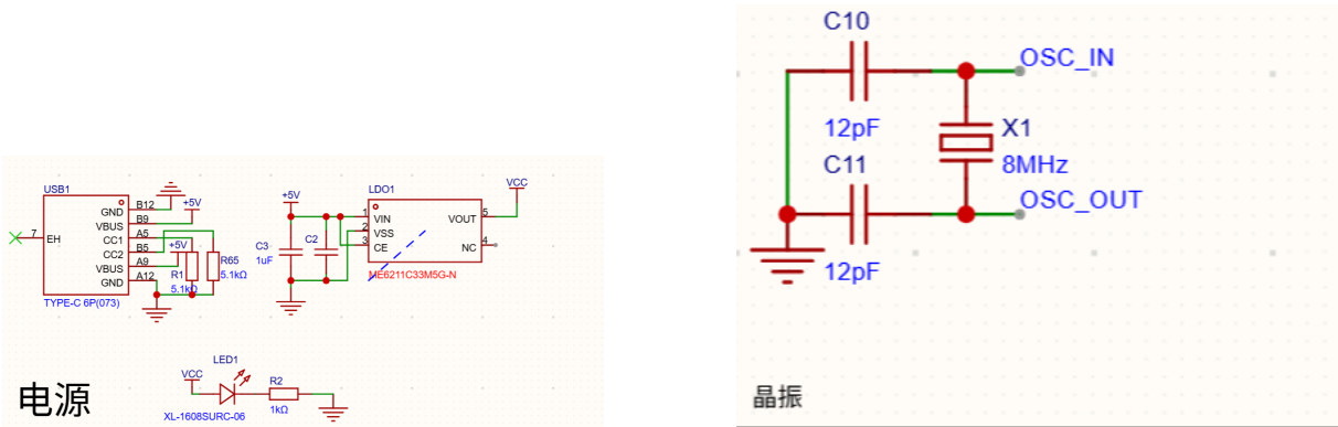
图 4-7 电源芯片（左）与时钟电路（右）
