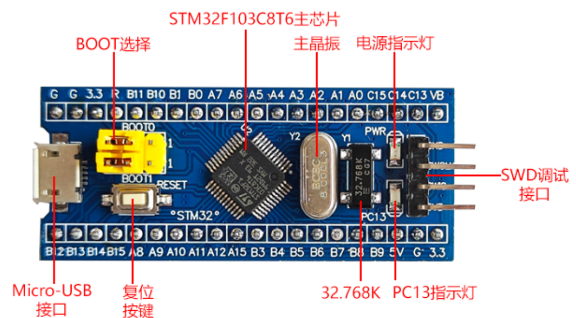
图 4-1 STM32F103C8T6 芯片实物图
