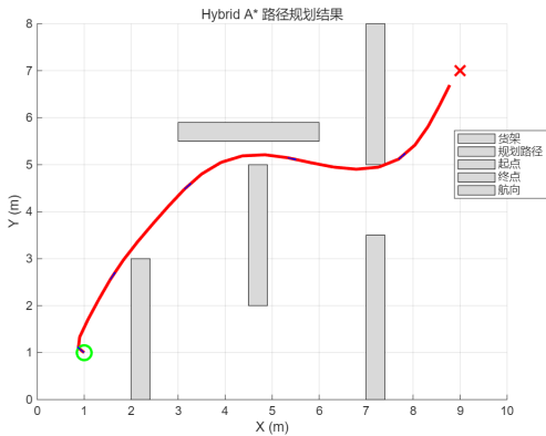
图 5-10 Hybrid A* 路径规划结果
