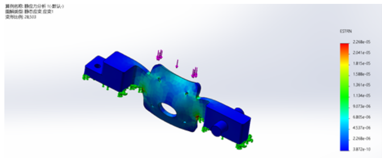
图 3-6 支撑梁最大应变分布示意图
