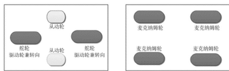
图 2-3 全方位驱动示意图
