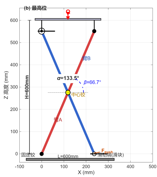
图 3-4 剪叉式升降机构运动简图（最高位）
