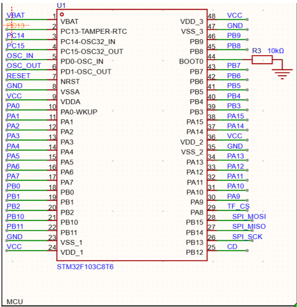
图 4-2 STM32F103C8T6 芯片示意图
