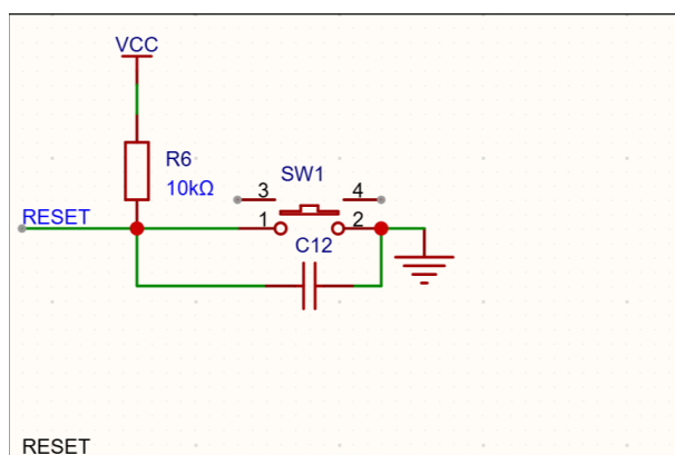
图 4-11 复位电路示意图
