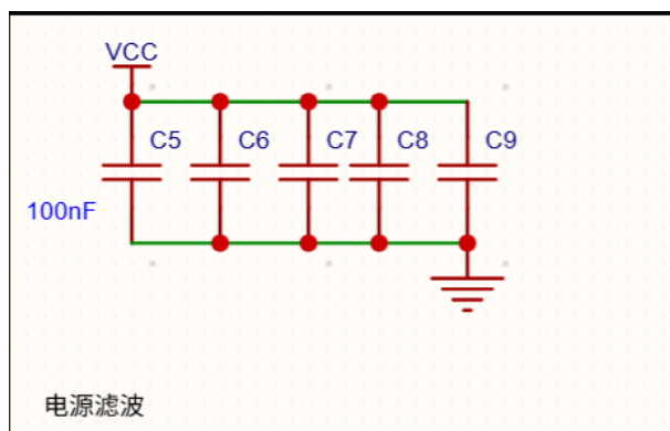
图 4-8 电源滤波电路示意图
