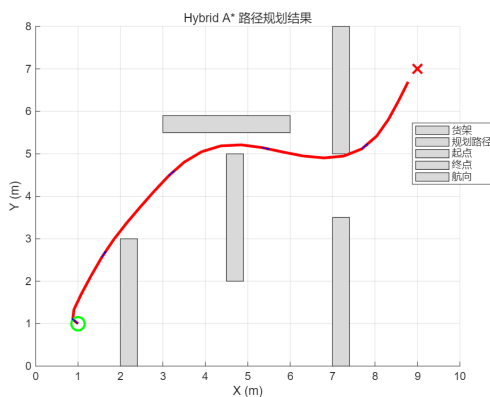
图 5-10 Hybrid A* 路径规划结果
