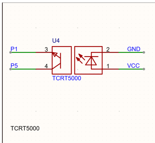
图 4-12 红外线传感器接口电路示意图
