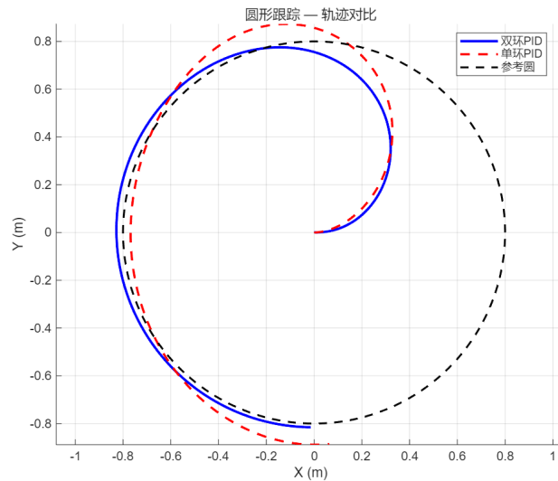
图 6-8 圆形轨迹跟踪对比
