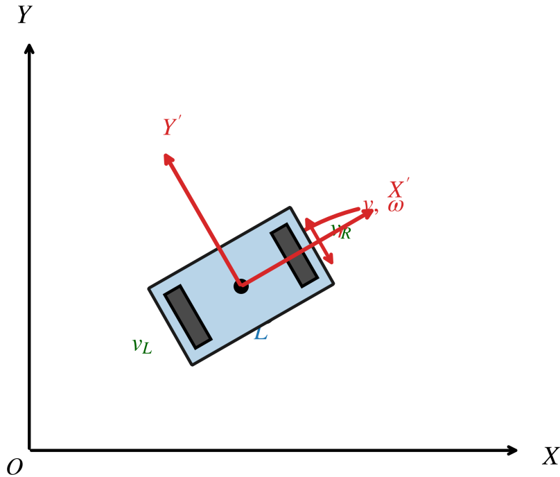
图 5-1 双轮差速移动机器人模型示意图
