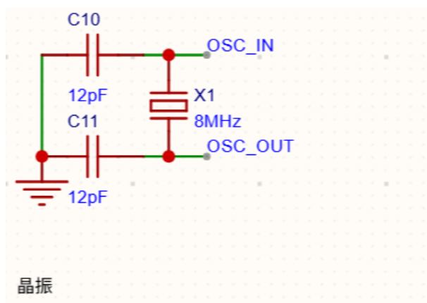
图 4-9 时钟电路示意图
