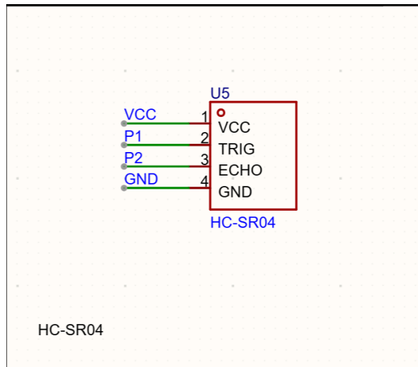
图 4-13 超声波传感器接口电路示意图
