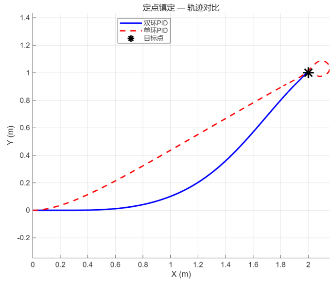
图 6-2 定点镇定轨迹
