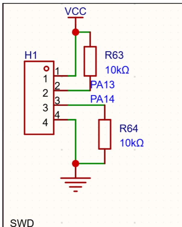
图 4-10 SWD 程序下载调试电路示意图
