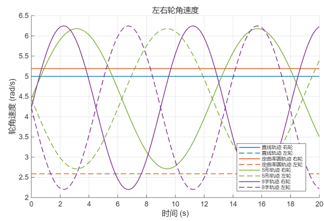
图 5-8 四类轨迹左右轮角速度
