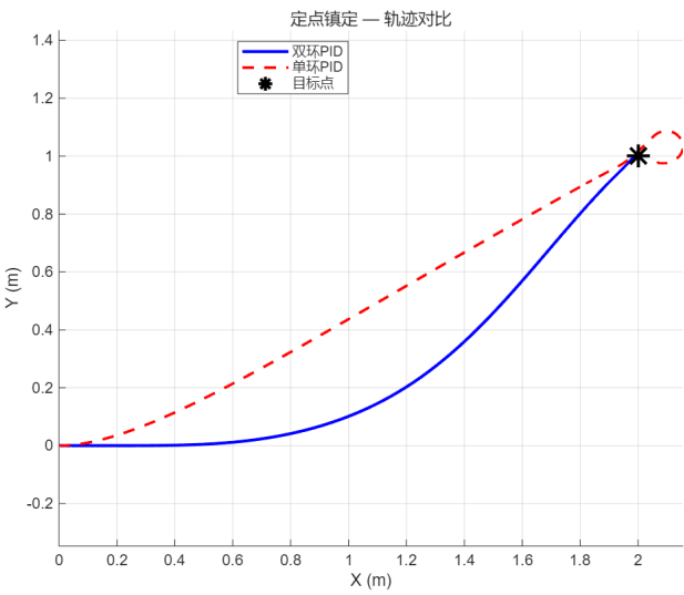
图 6-6 定点镇定轨迹对比
