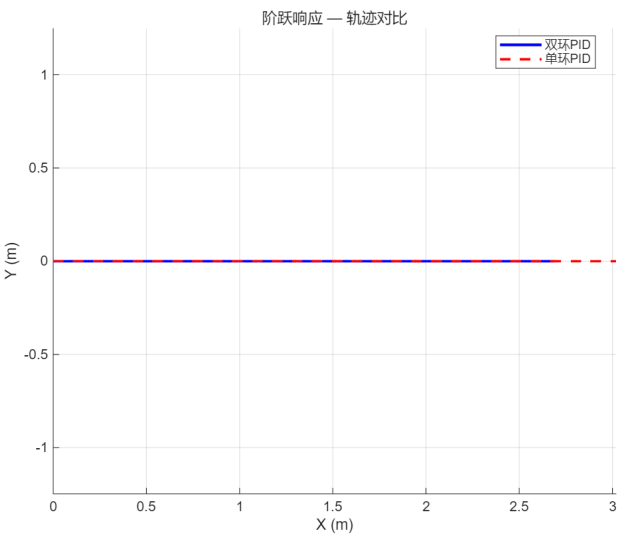
图 6-5 阶跃响应轨迹对比
