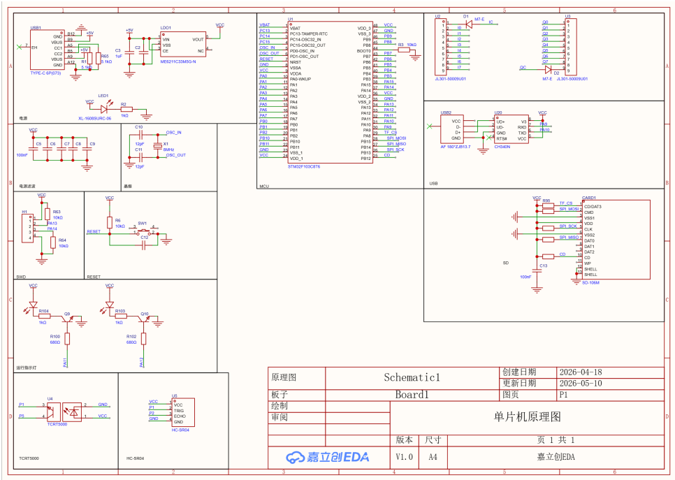
图 4-6 STM32F103C8T6 最小系统示意图
