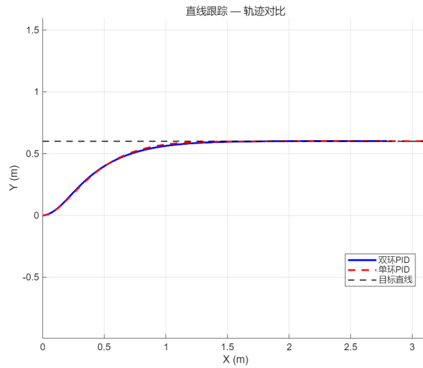
图 6-7 直线跟踪轨迹对比
