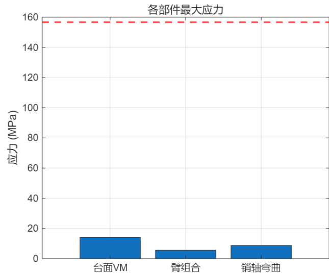
图 3-6 各部件最大应力对比
