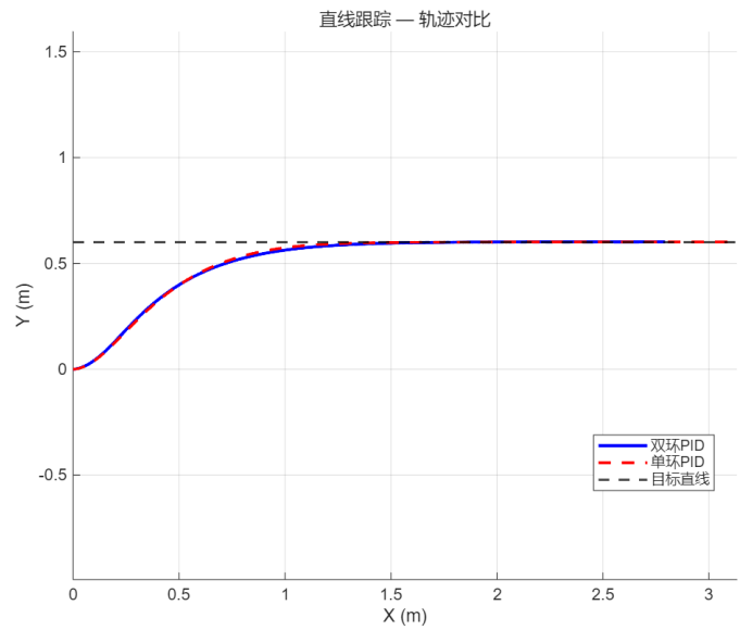
图 6-3 直线跟踪轨迹
