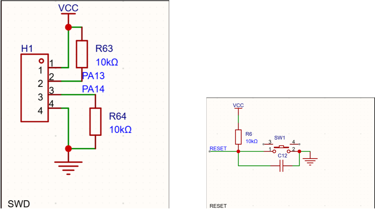
图 4-8 SWD 调试接口（左）与复位电路（右）
