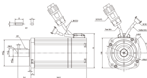
图 4-3 SMC80S-0040-30A 0 K-3DKH 伺服电机外形图
