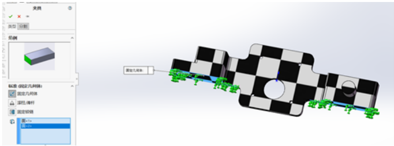
图 3-6 固定支撑梁的有限元分析示意图
