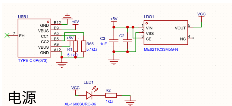
图 4-3 电源控制部分示意图
