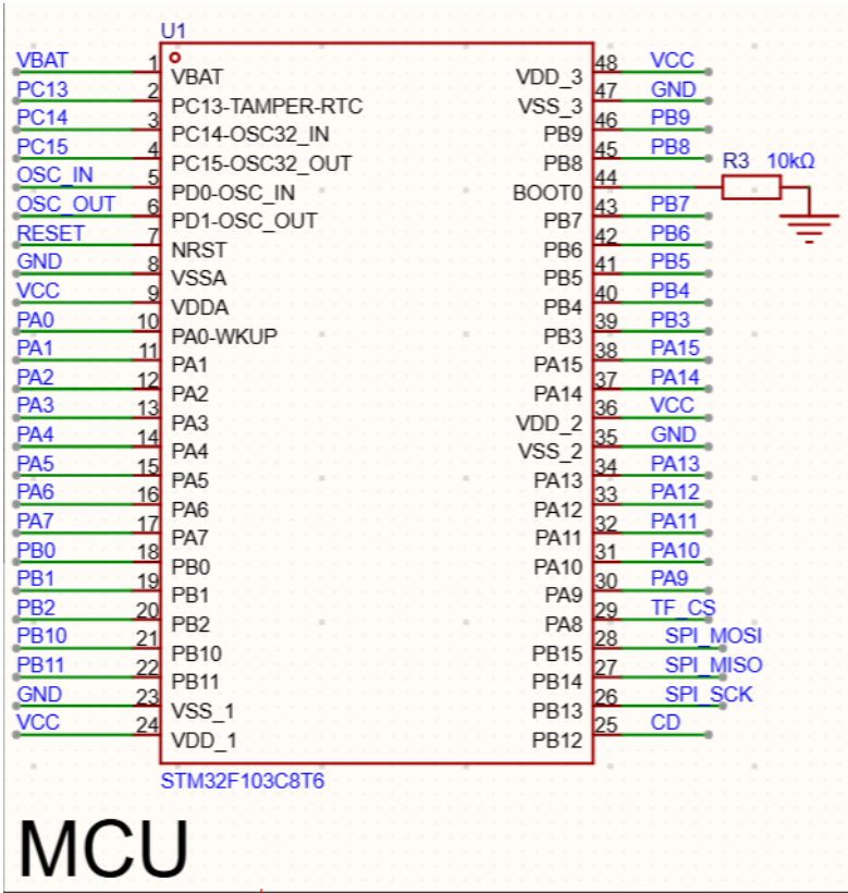
图 4-2 STM32F103C8T6 芯片示意图
