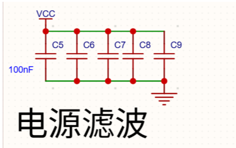
图 4-8 电源滤波电路示意图
