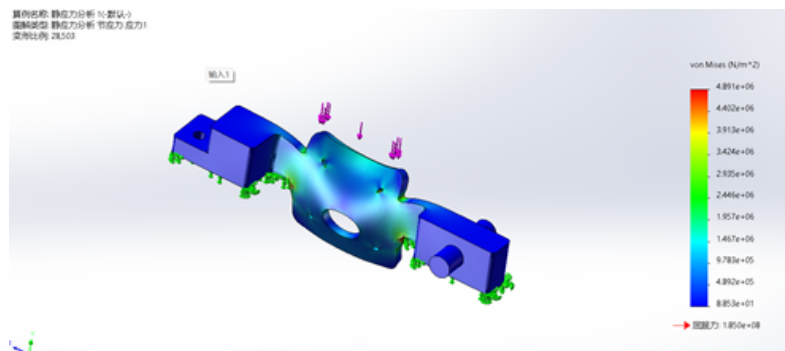
图 3-8 支撑梁受力仿真结果示意图
