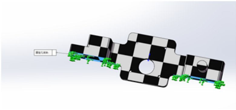
图 3-5 固定支撑梁的有限元分析示意图
