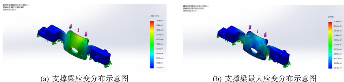
图 3-9 支撑梁应变分析结果对比图
