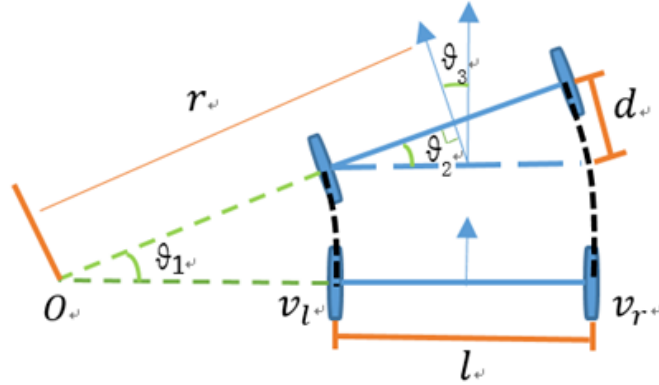
图 5-1 双轮差速移动机器人模型示意图
