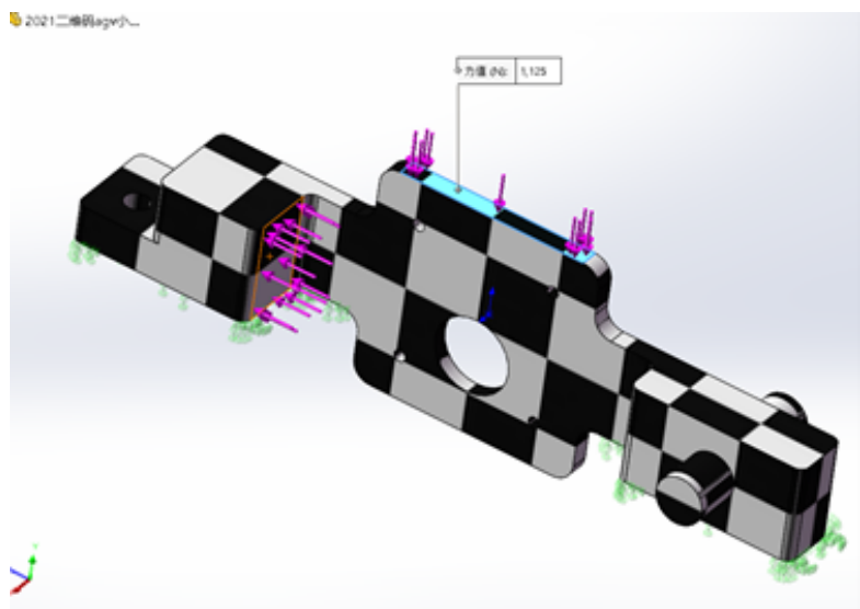
图 3-6 施加受力的有限元分析示意图
