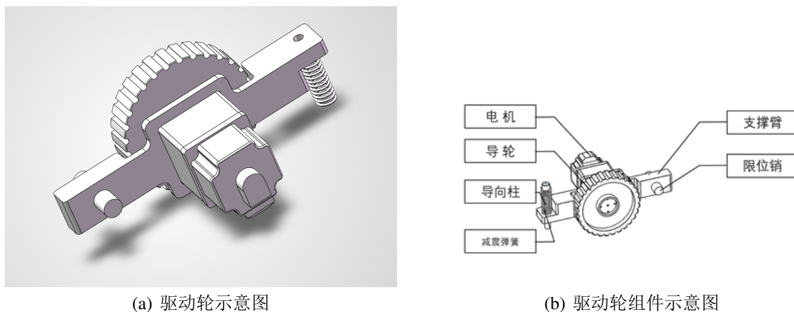
图 3-2 驱动轮及组件示意图
