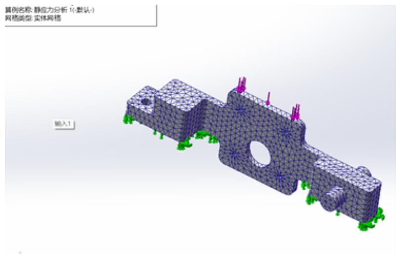
图 3-7 支撑梁的网格划分示意图
