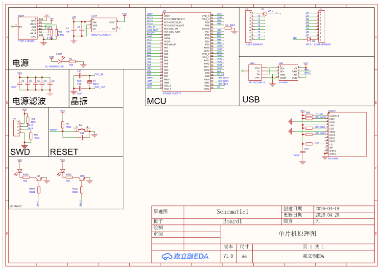
图 4-7 STM32F103C8T6 最小系统示意图
