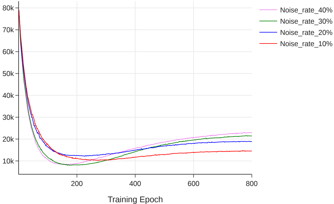
Dirichlet Energy
