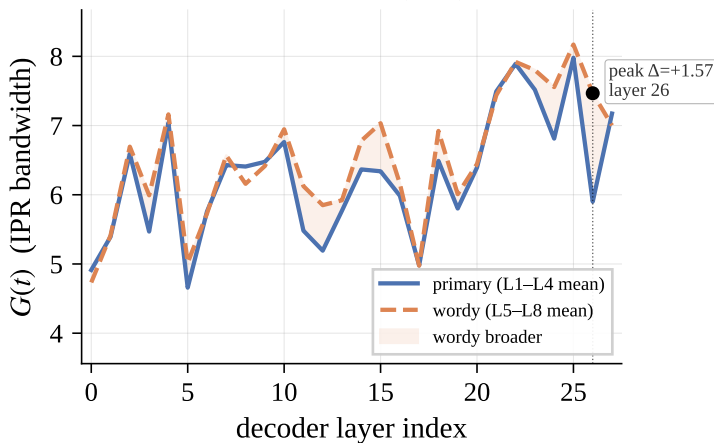
CLEVR-2B (B=9)
